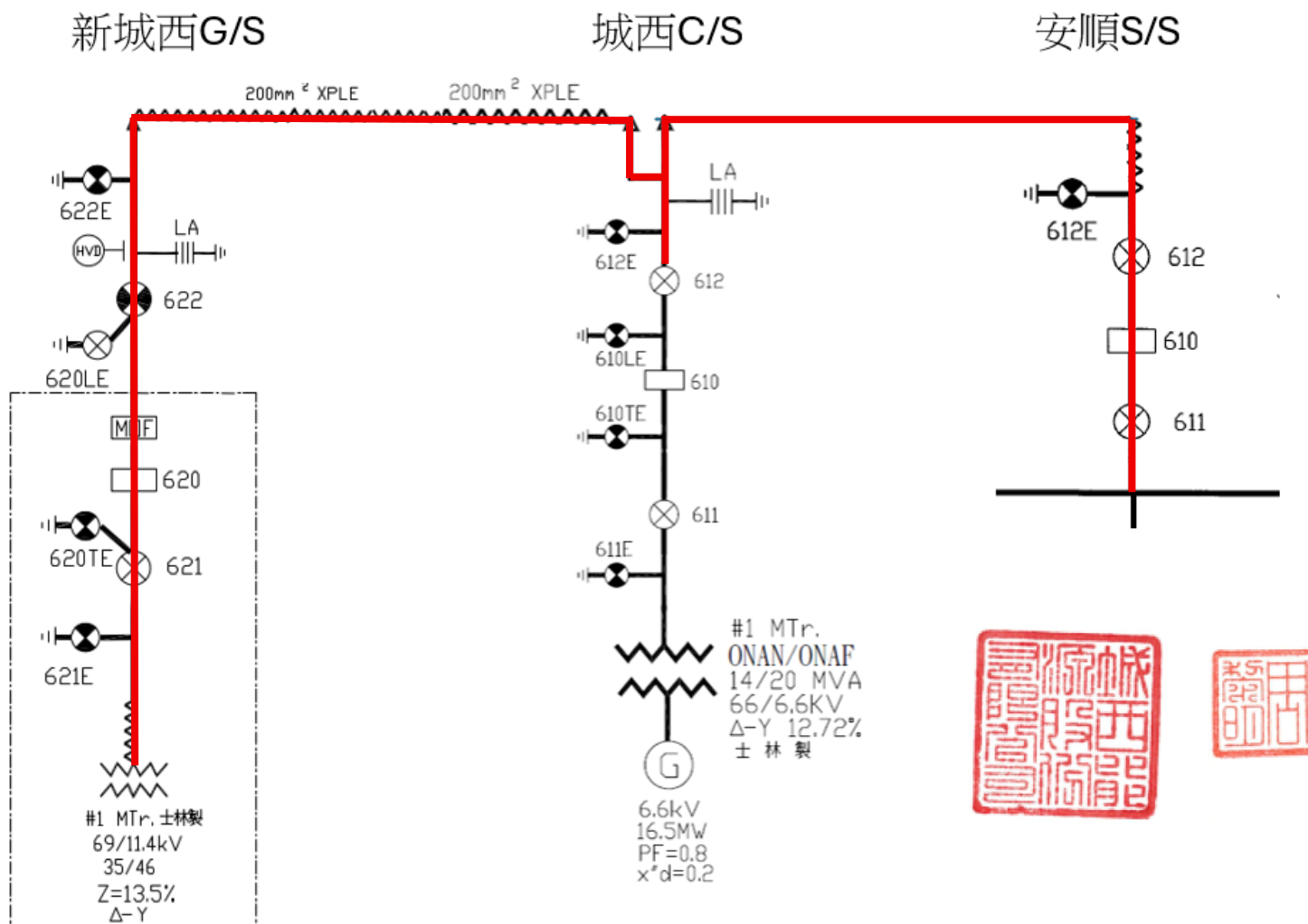
圖一、(新城西 G/S)加壓示意圖：
